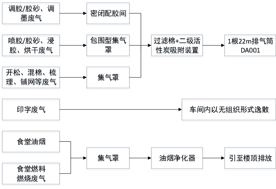
图 4.5-2 项目废气收集及治理措施汇总图
